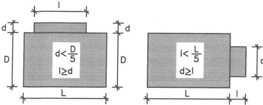
الف) پیش‌آمدگی در امتداد طول ساختمان ب) پیش‌آمدگی در امتداد عرض ساختمان
